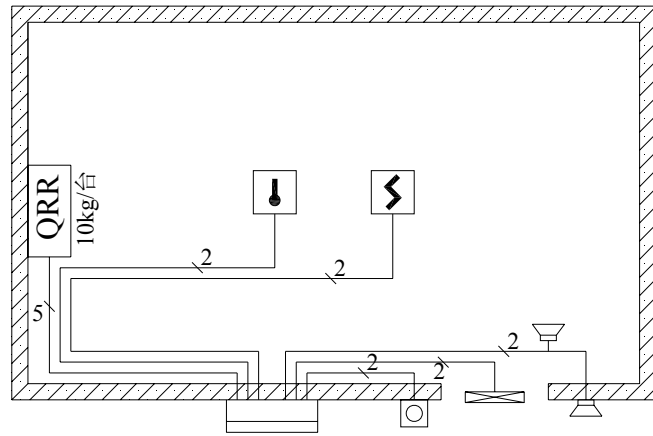
图例： QRR 热气溶胶灭火装置 2 连线数 灭火控制器 喷放指示灯 感温探测器 紧急启动按钮 感烟探测器 声光报警器
