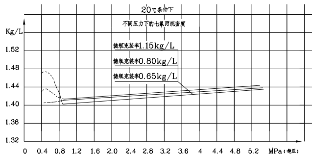
图 3.3.15-2 不同压力下七氟丙烷的密度
