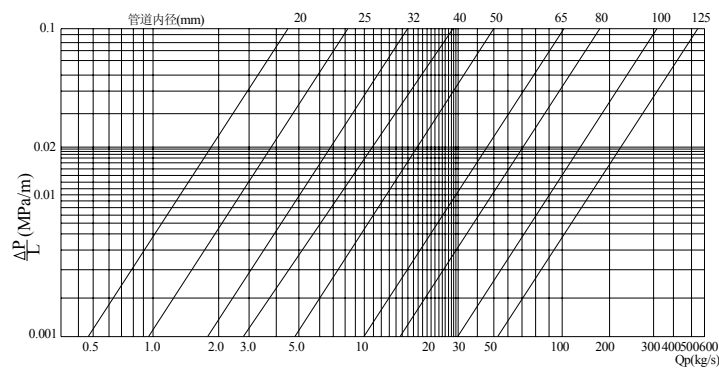
图 3.3.15-1 镀锌钢管阻力损失与七氟丙烷流量的关系
